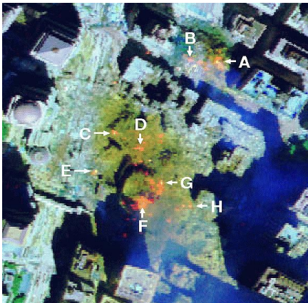
Värmebilder tagna från satellit av NASA den 16:e september visar yttemperaturer på upp till 800°C
